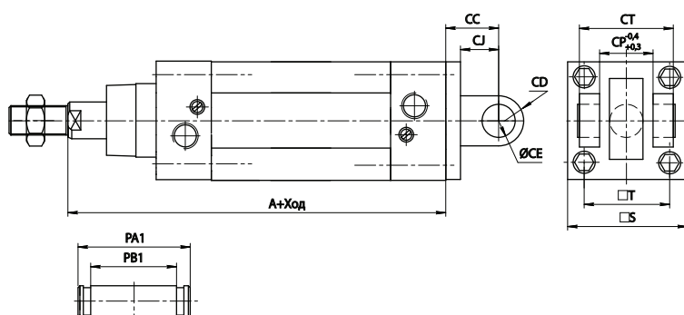
Шарнирное крепление под углом 90° для серий SR, SE. Код: SC-SE/SR-CR-(диаметр)
