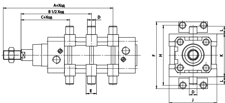
Центральная подвеска для серии SE. Код: SC-SE/SR-TC-(диаметр)
