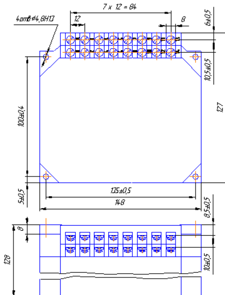
Рисунок 2 - Габаритные и установочные размеры реле ВС44-3, ВС44-4
