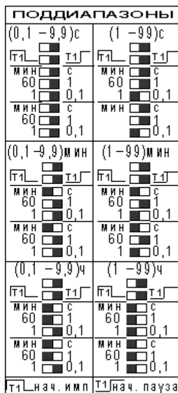
Рисунок 3 - Положение переключателей диапазонов (установка поддиапазонов выдержек времени)
