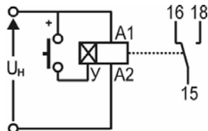
Рисунок 2 - Схема подключения реле.
